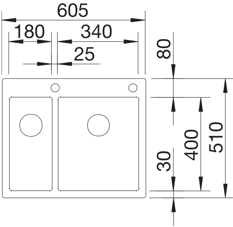
Aufsicht
